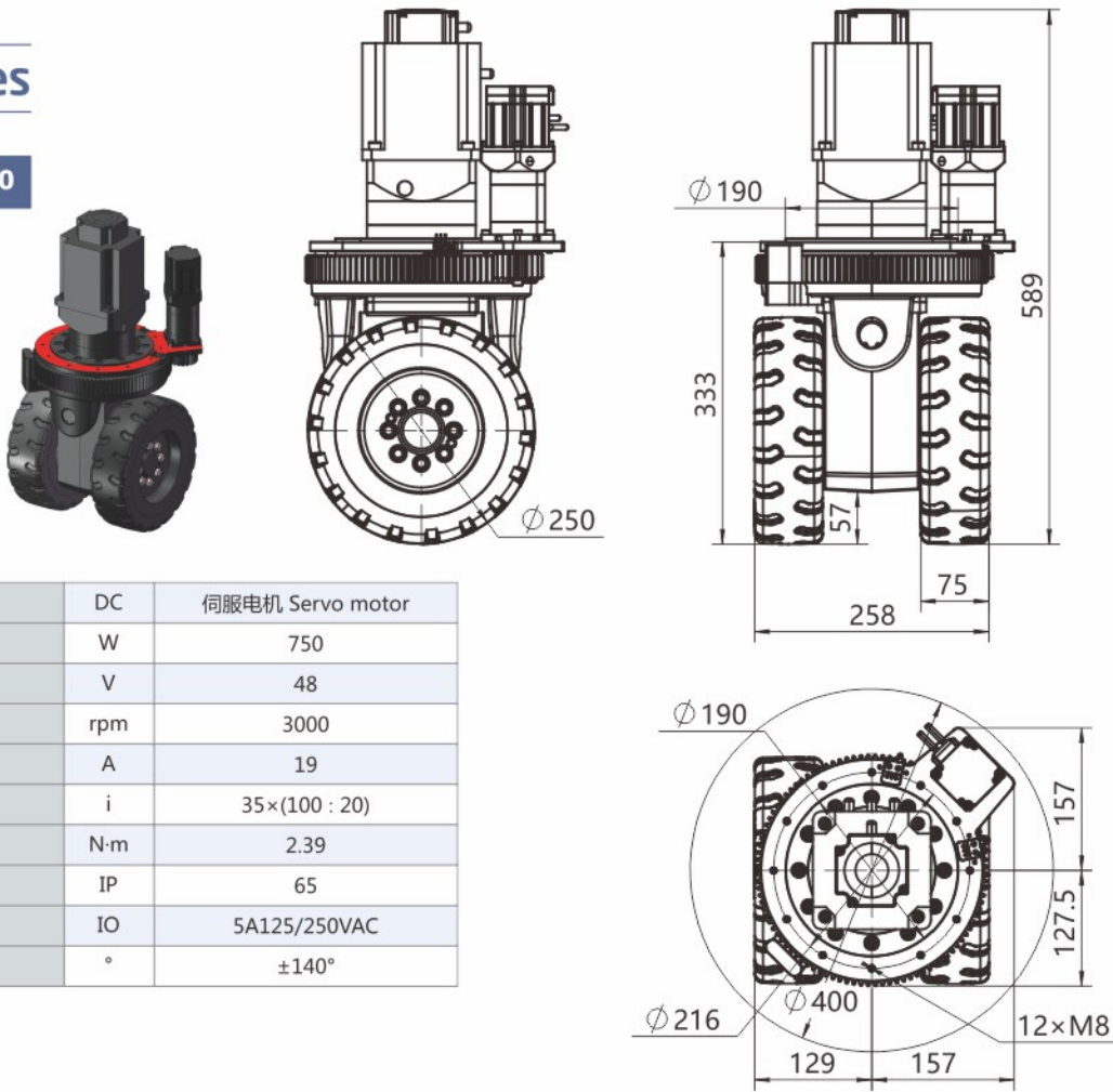
牵引电机参数 Parameters of traction motor
