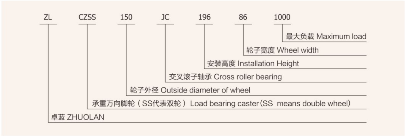
CZSS系列型号说明 CZSS series model description
