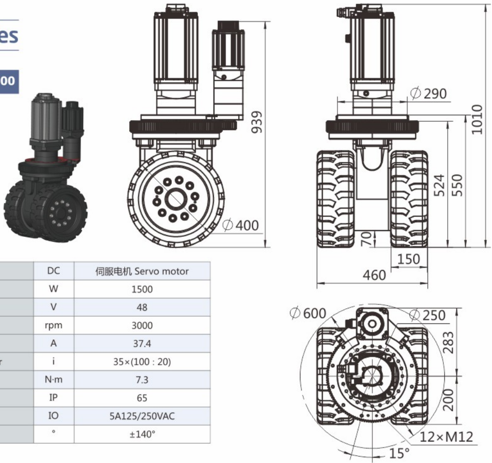
转向电机参数 Steering motor parameters
