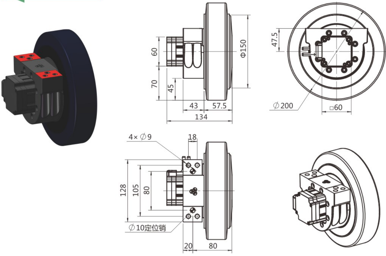
牵引电机参数 Parameter list of traction motor
